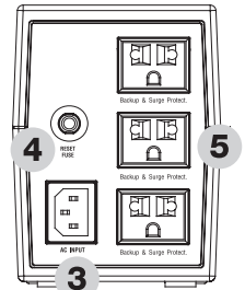
หลังเครื่อง 3. AC Input 4. Reset Fuse 5. AC Output & Surge Protection
